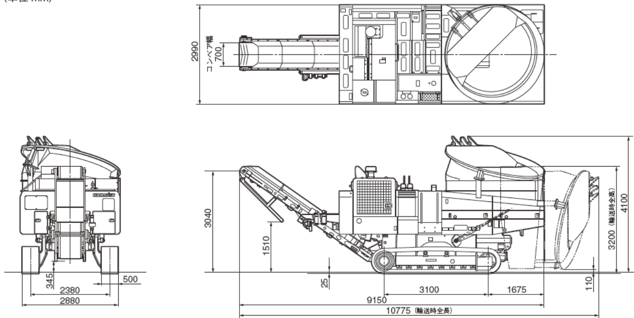
外形図 (単位:mm)
