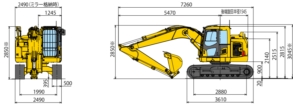
PC138US-11 トンネル仕様 (4.6mブーム、2.5mアーム)
