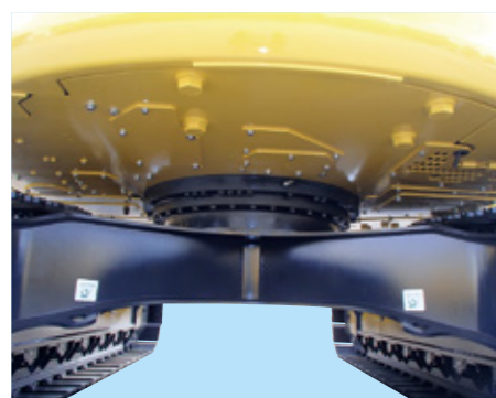
レボフレーム強化アンダーカバー (写真はPC138US-11)
