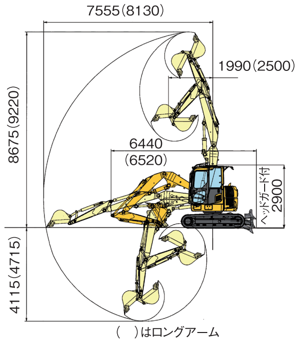
PC78US-10
