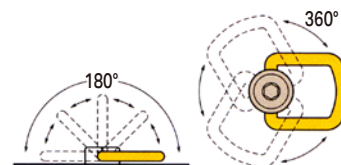
<B型> JISアイボルト対応タイプ SYOH-B□□
