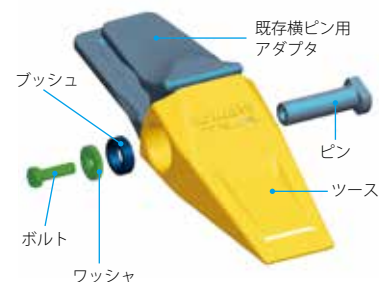
ハンマレス PAB ツースシステム (Pin And Bushing System)
